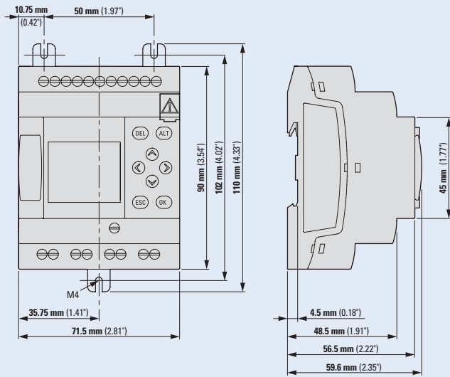
Základní přístroj s displejem
