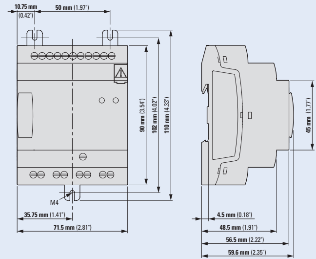
Základní přístroj bez displeje
