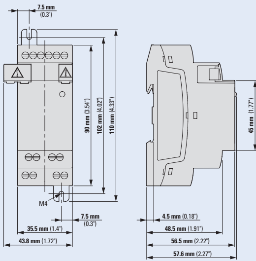
Malý rozšiřující modul
