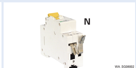
Připojovací úhelník ZV-N0,5TE pro N vodič 0,5 TE (např. pro PL7...1,5 TE)
