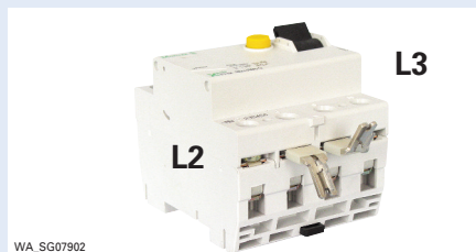
Připojovací úhelník ZV-L2/L3 pro L2 a L3
