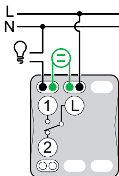
Jednopólové ovládání zap/vyp s orientační kontrolkou
