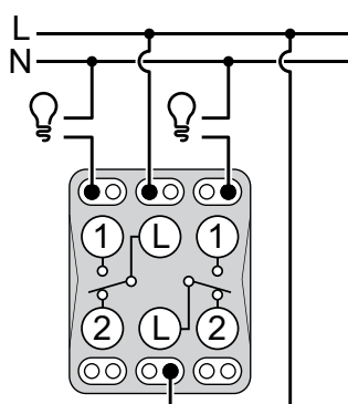
Dva jednopólové zap/vyp spínání
