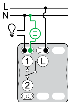
Jednopólové ovládání zap/vyp se signalizační kontrolkou
