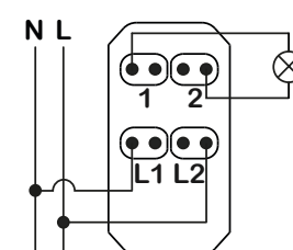
Dvopolový spínač
